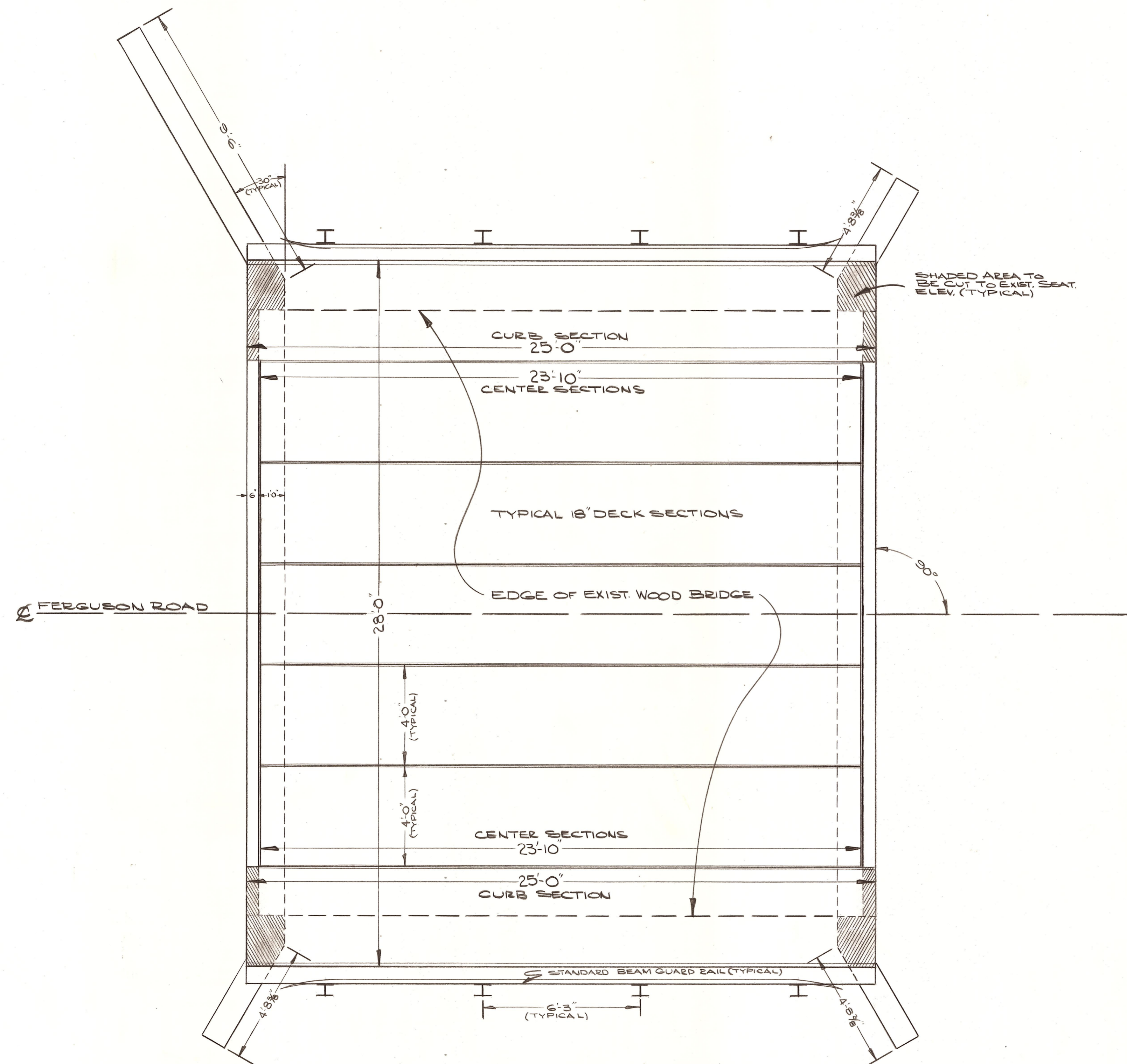
PLAN SCALE: 3/8"=1'-0"
